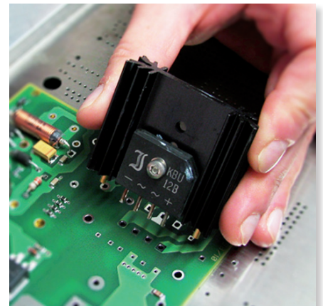
Abb. 2: THT-Bestückung
