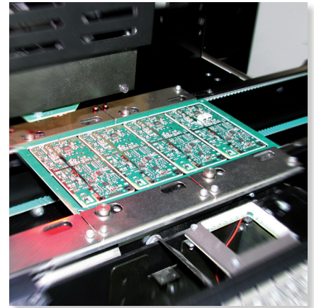
Abb. 1: SMD-Linie
